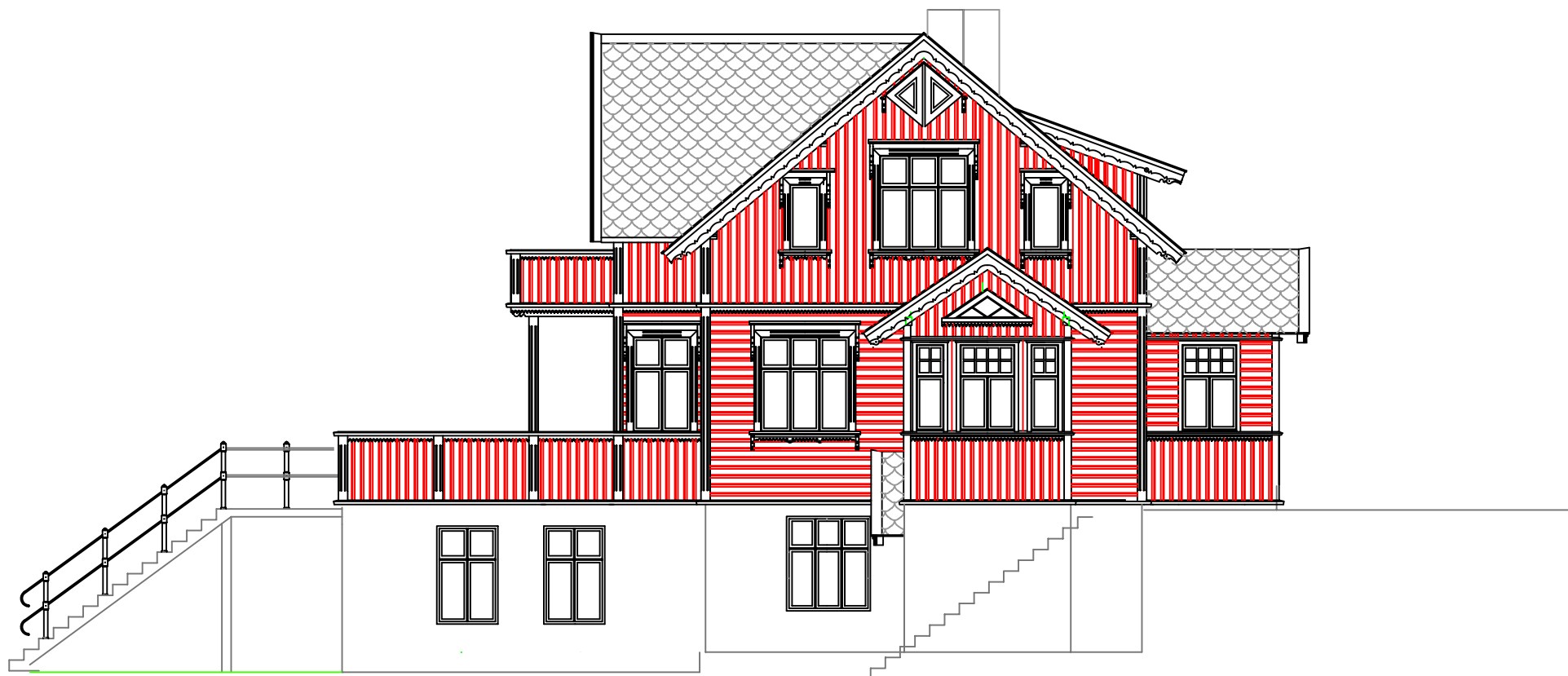
FASADE MOT AUST
