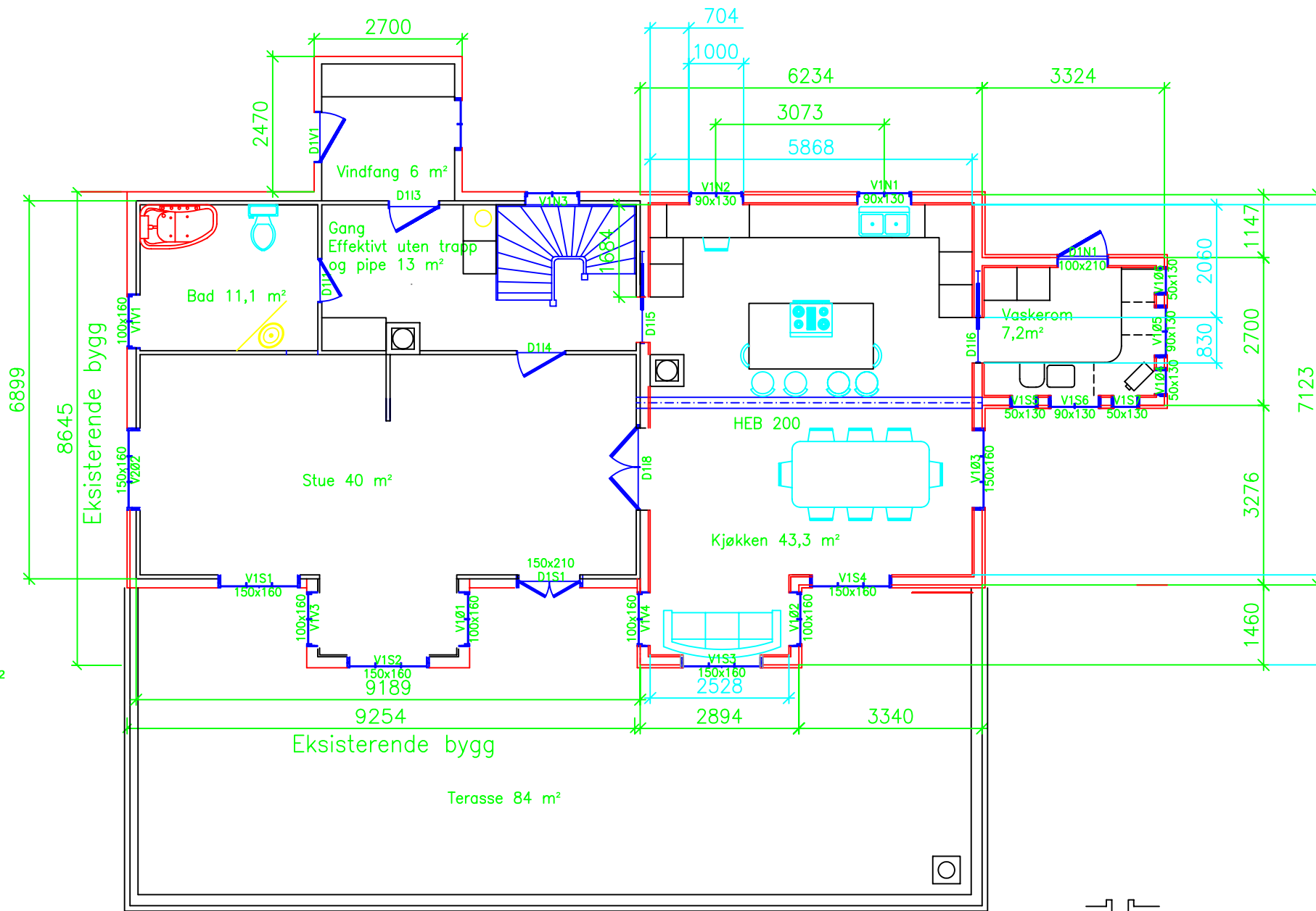
PLAN 1 ETG.
